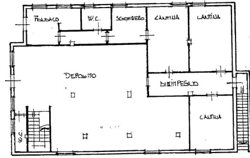
PIANTA PIANO SEMINTERATO H= 2.50
